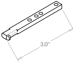
Barre de pivot G1-42-PB62-00
