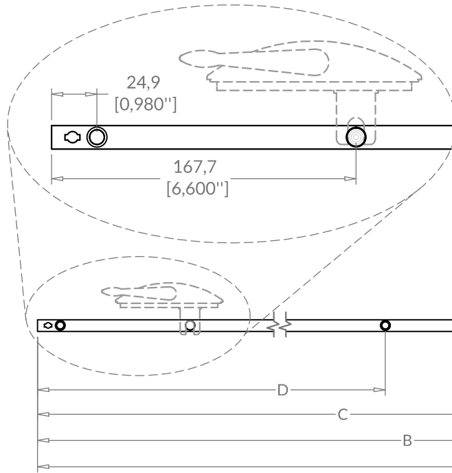
DÉTAIL A (ÉCHELLE 2:1)
